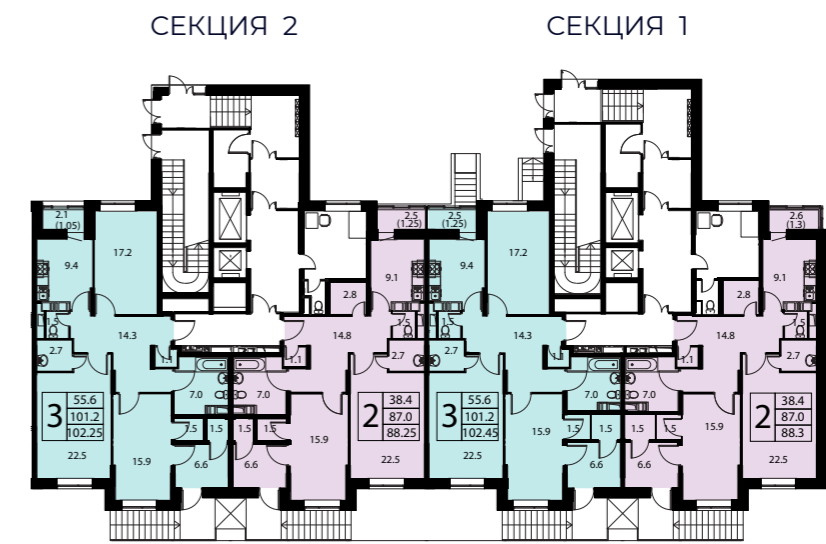
ЭТАЖ 1
