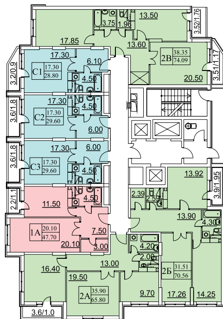
Корпус 3, секция 4-5 17-18 этажи
