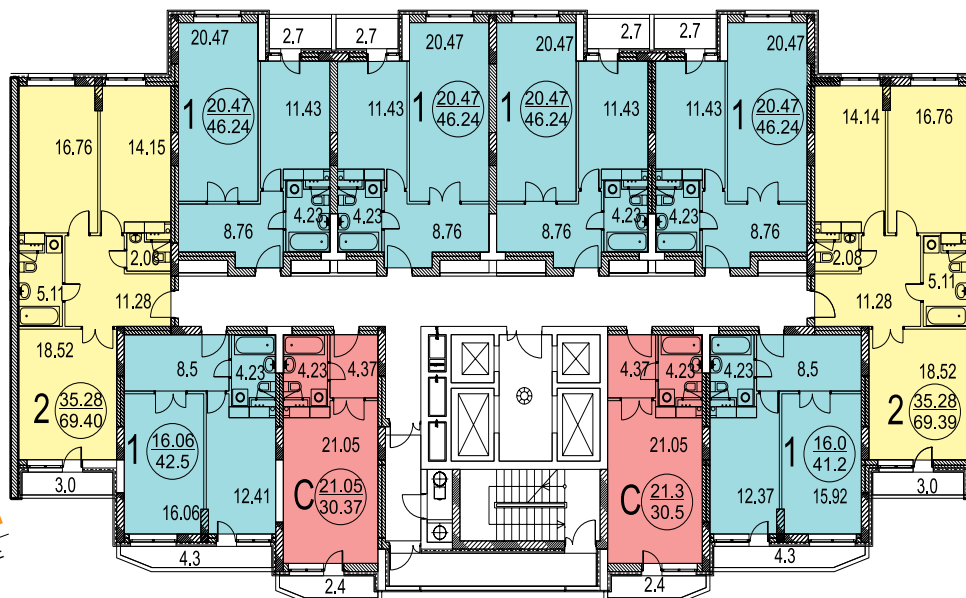
Корпус 1, секция 2, ТИПОВОЙ ЭТАЖ
