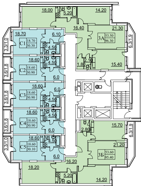
Корпус 3, секция 4 19-25 этажи
