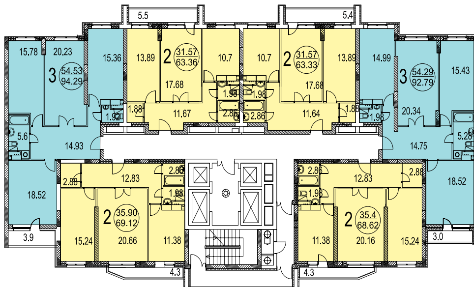
Корпус 1, секция 2, ТИПОВОЙ ЭТАЖ
