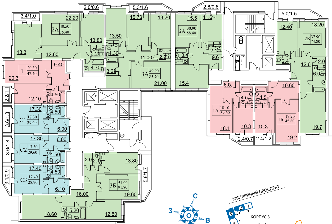
Корпус 3, секция 2-3 17-18 этажи
