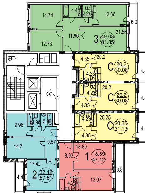
Корпус 1, секция 6, 2-5 этажи
